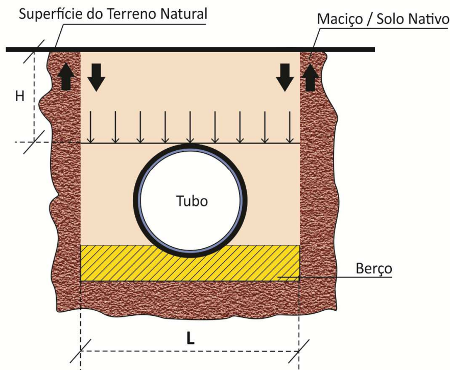
Figura 28 - Carga de solo atuante.
