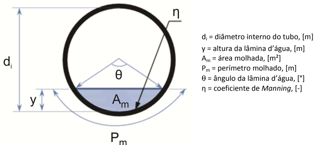
Figura 31 - Variáveis para dimensionamento hidráulico
