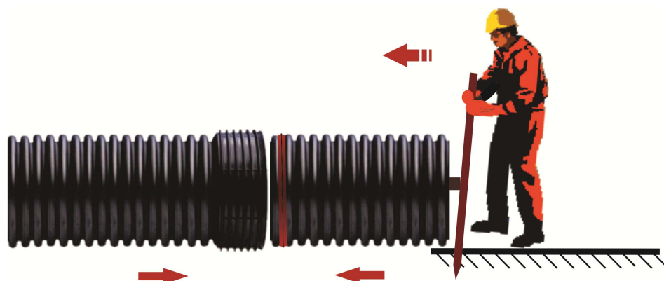
Figura 35 - Introdução da ponta na bolsa
