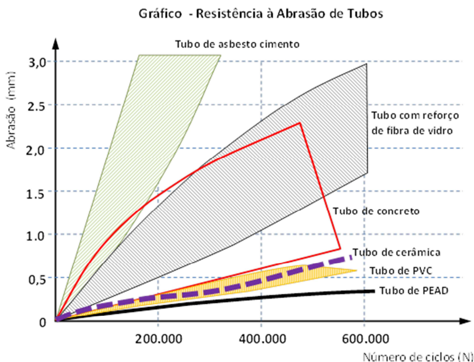
Figura 3 - Gráfico de Abrasão (DIN 19534) - Universidade de Darmstadt
