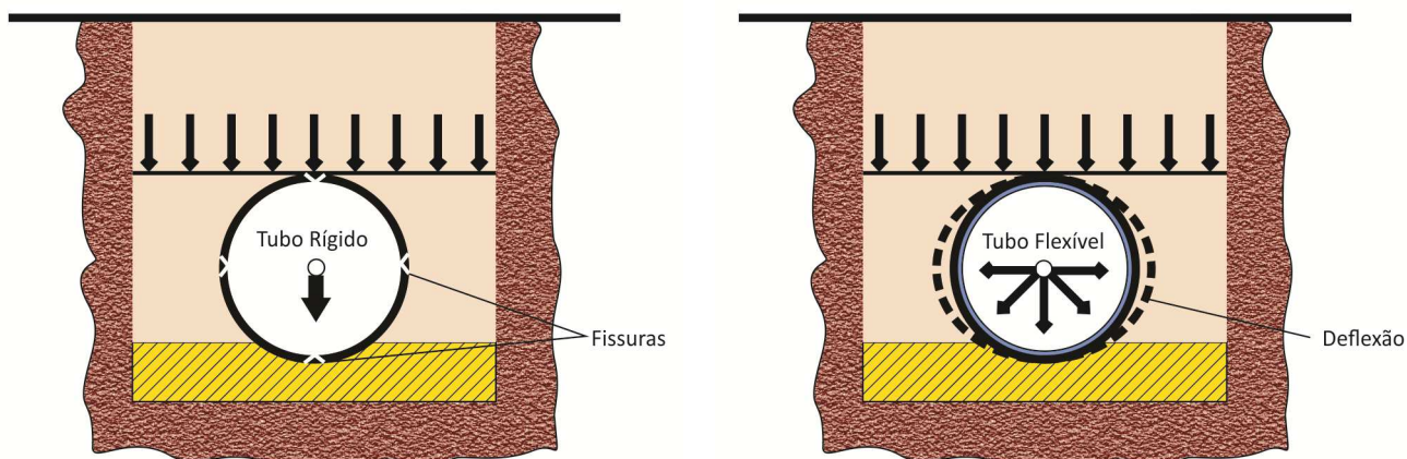
Figura 23 – Comportamento dos tubos sob ação de carga vertical
