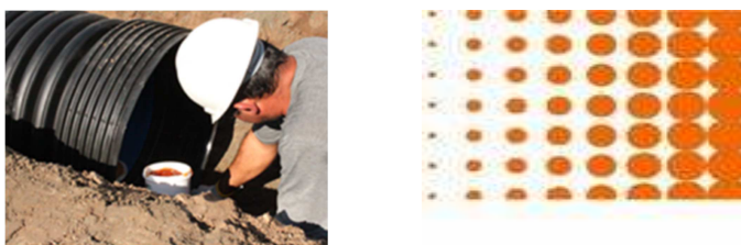
Figura 33 - Aplicação da pasta lubrificante
