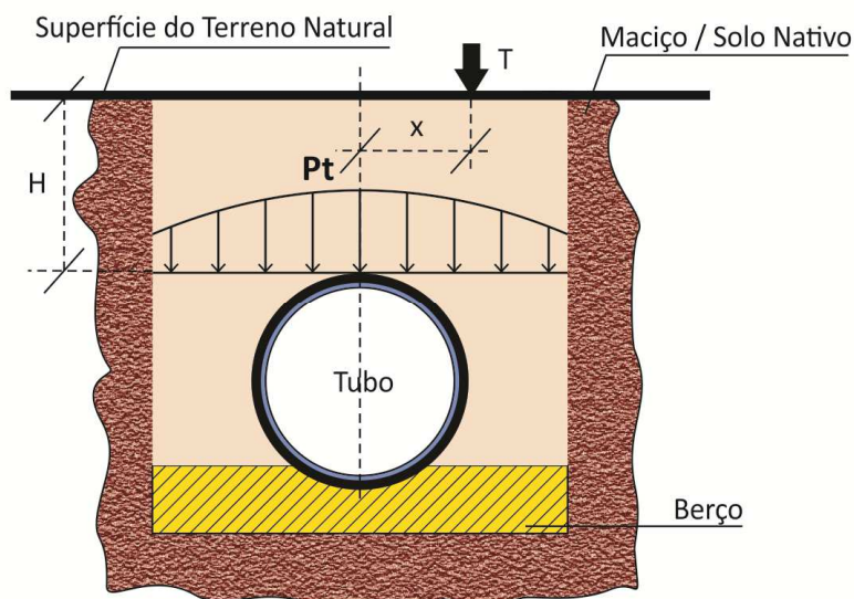
Figura 29 - Carga de tráfego
