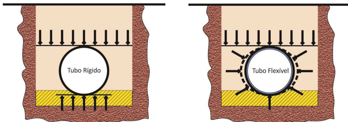
Figura 24 – Interação Solo / Tubo (tubo com o solo de envoltória)
