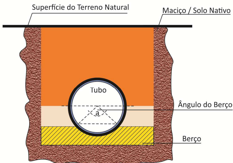
Figura 30 – Ângulo do berço
