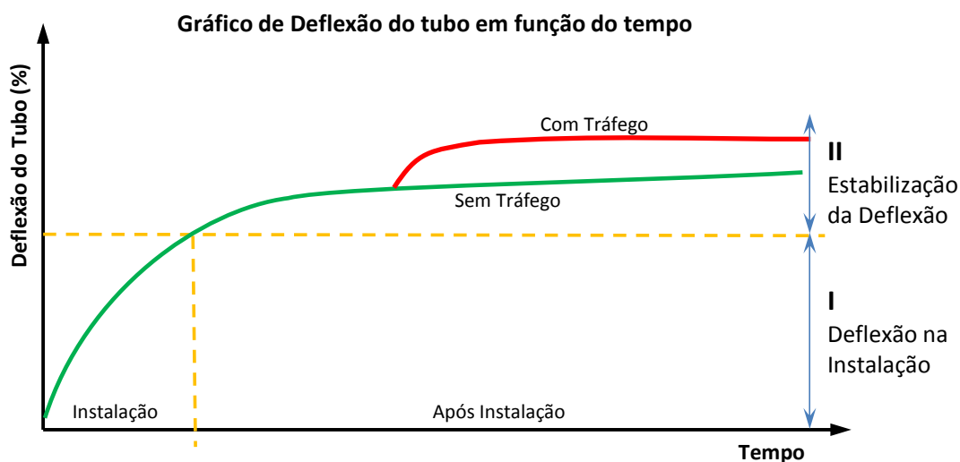
Figura 27 - Gráfico de deflexão do tubo no momento da instalação e após sua instalação
