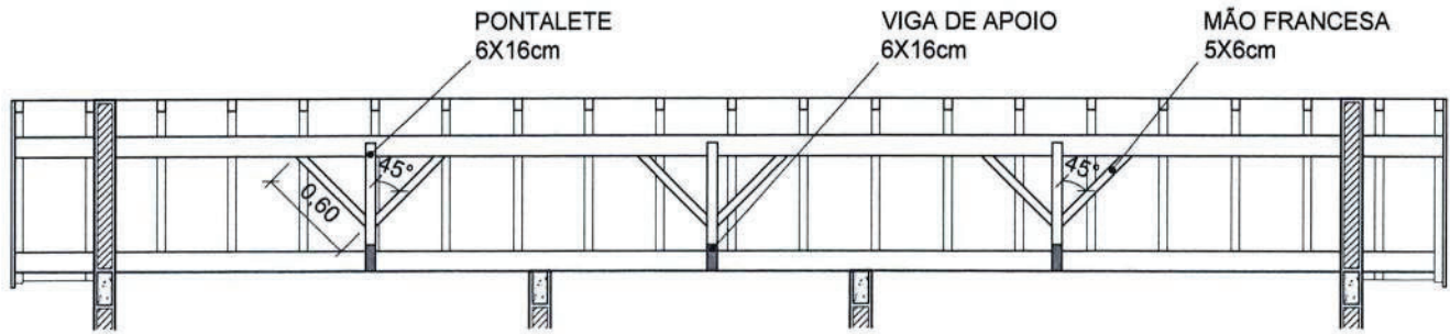
CORTE EE
