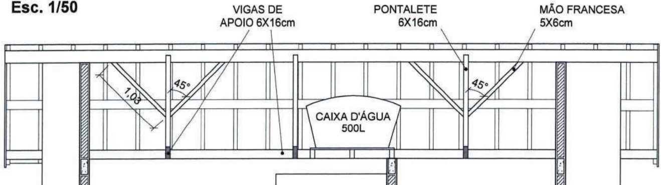
CORTE FF
