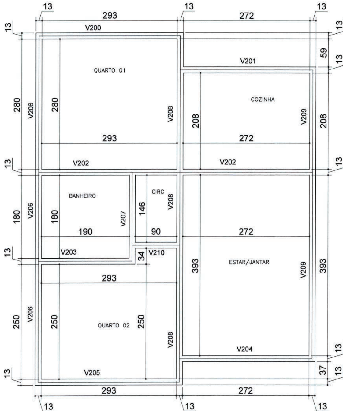
PLANTA DE FORMA - VIGAS DE RESPALDO Esc. 1/50
