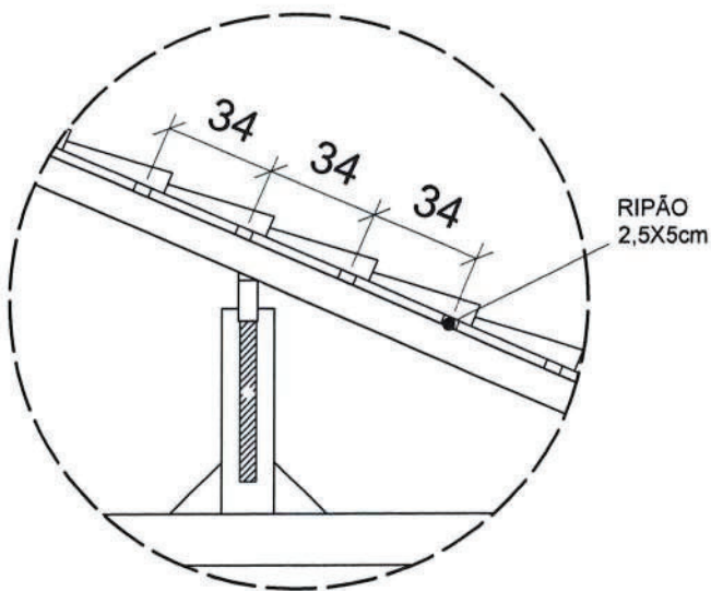
DETALHE 01 - RIPÃO
