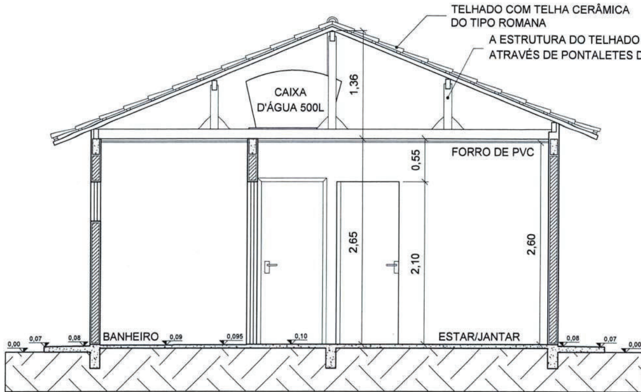
CORTE CC Esc. 1/50
