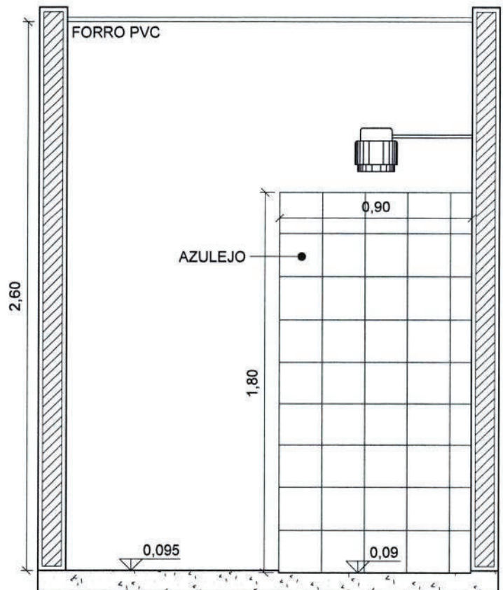
VISTA C Esc. 1/25
