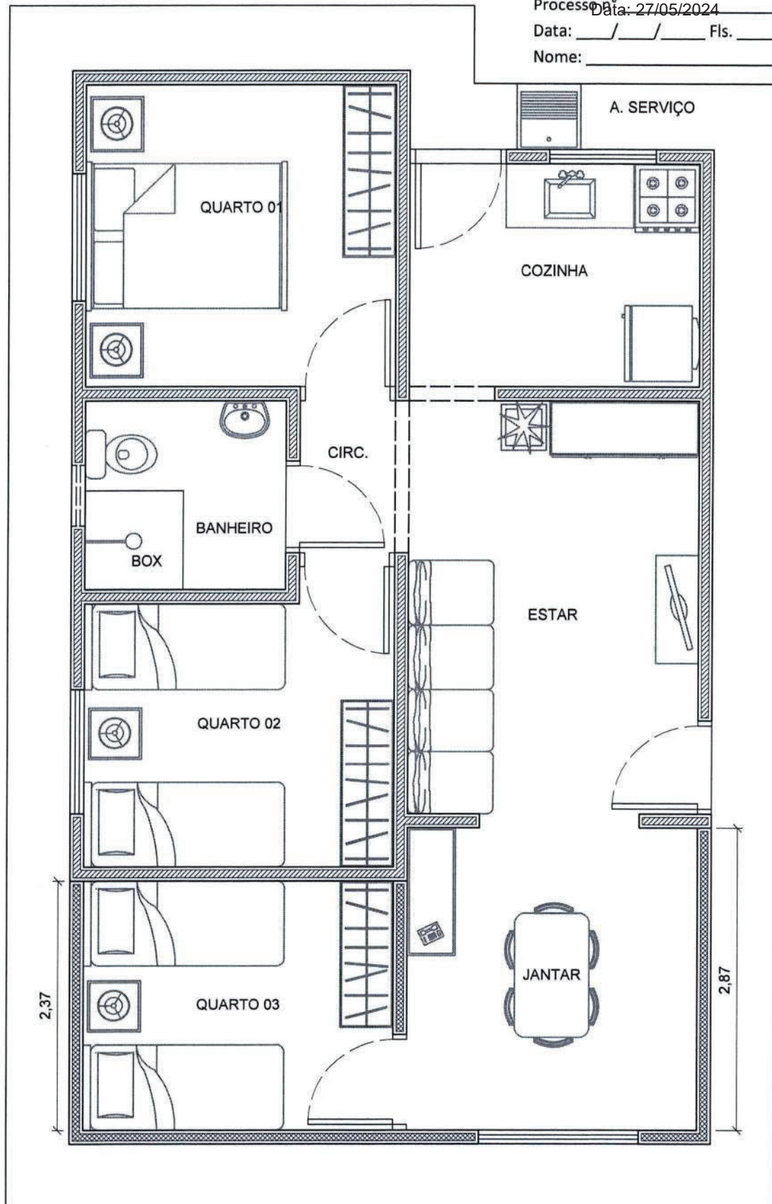
PLANTA AMPLIAÇÃO Esc. 1/50
