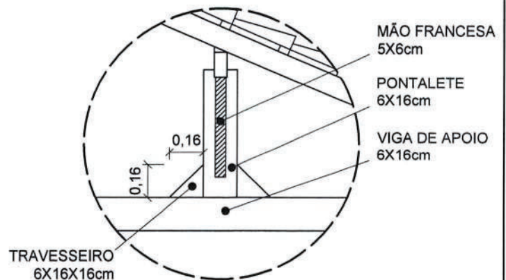
DETALHE 02 - PONTALETE
