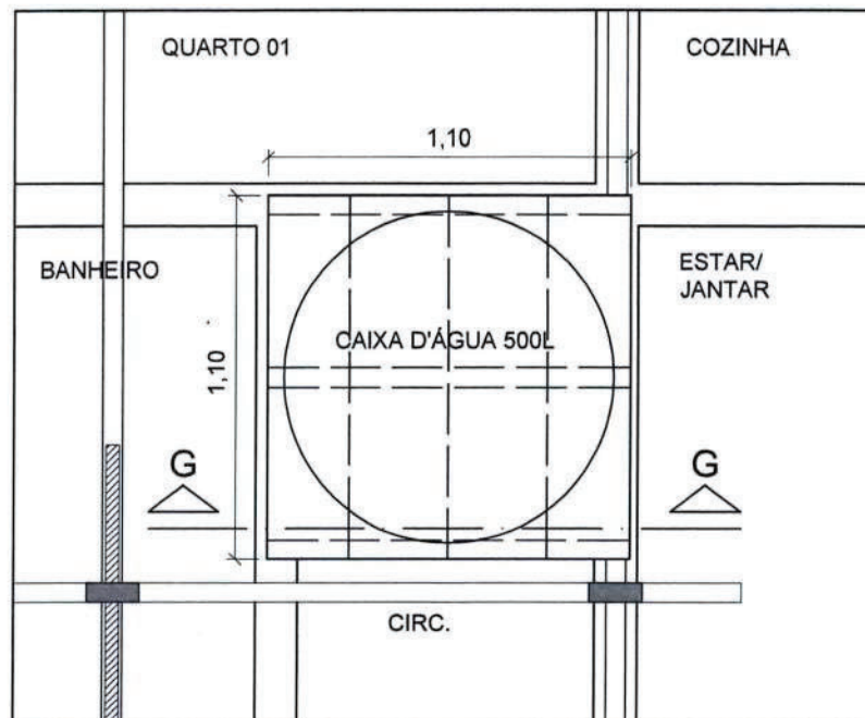
PLANTA - CX. D'ÁGUA Esc. 1/25
